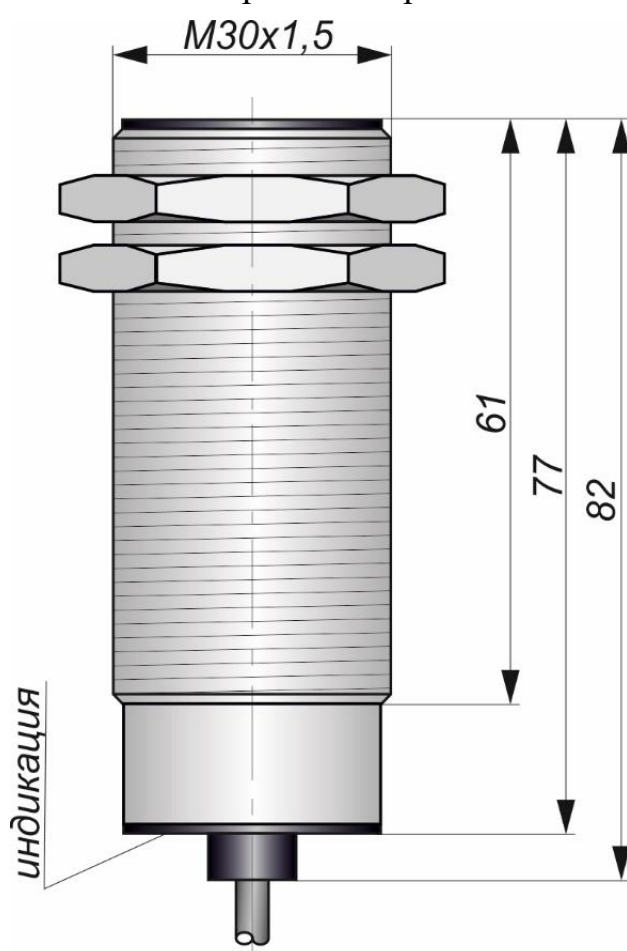
Габаритный чертеж
